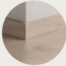
FARBlich PASSENDE STANDARD-SOCKELLEISTE 2400 x 12 x 58 mm PGSK(-)
